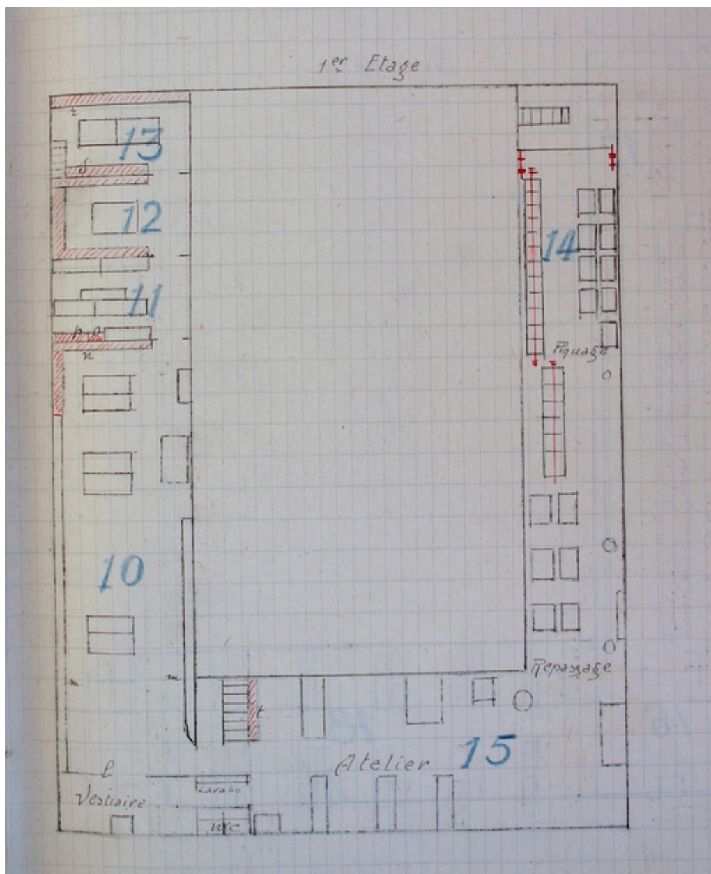
Plan du 1er étage des ateliers en 1914 (AD Aisne).
