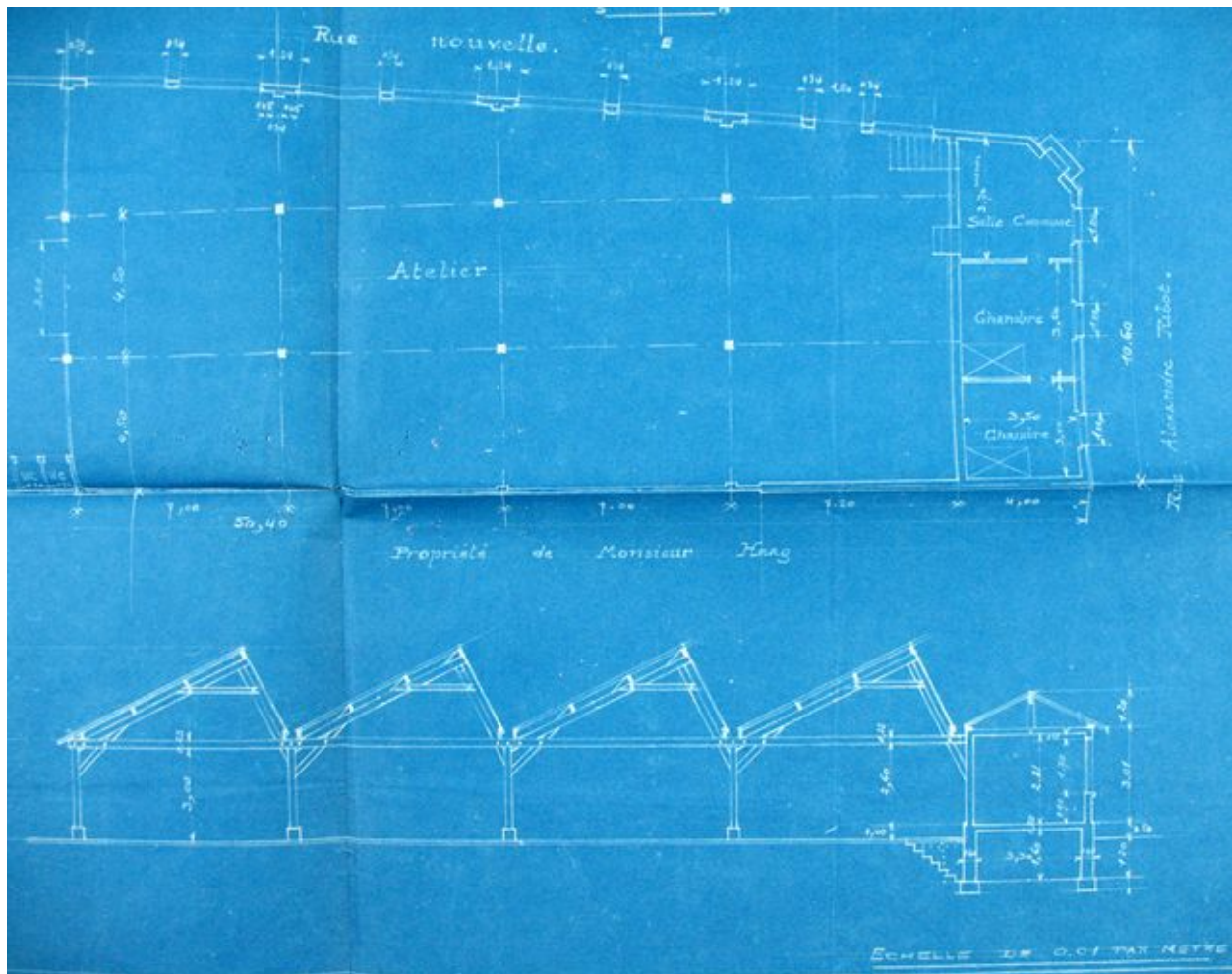
Plan de l'atelier de menuiserie mécanique, 1923 (AD Oise ; 5Mp2519).
