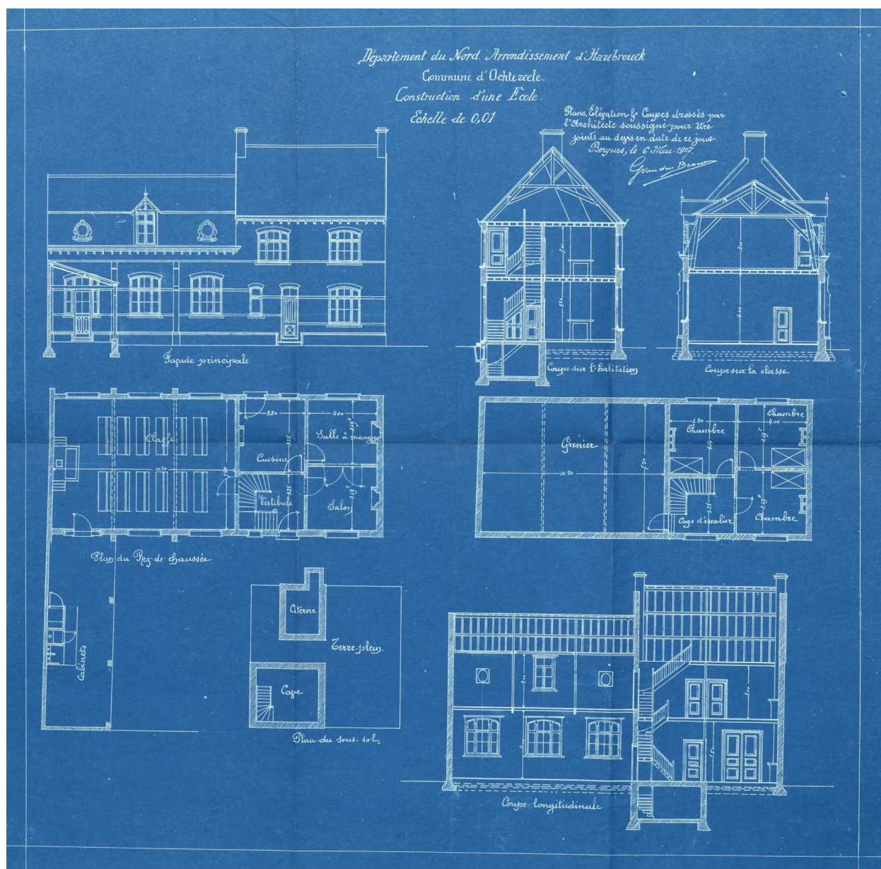
Plan, élévations et coupes - école d'Ochtezeele. Architecte : Van de Broeck. 6 mai 1907 (AD Nord 2 O 444/26).
