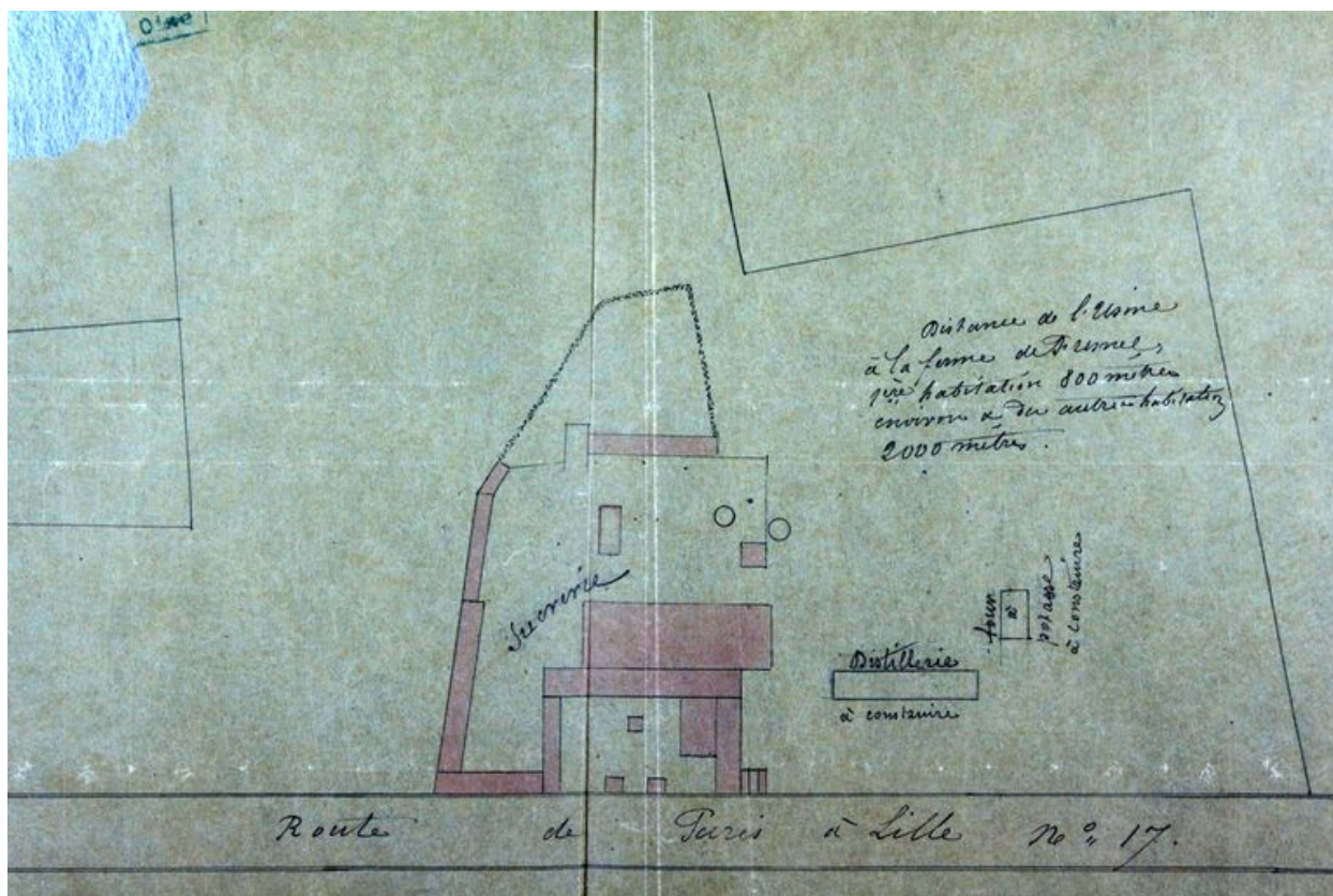
Plan masse de la sucrierie avec indication de la distillerie à construire, vers 1880 (AD Oise ; Mp 2474).
