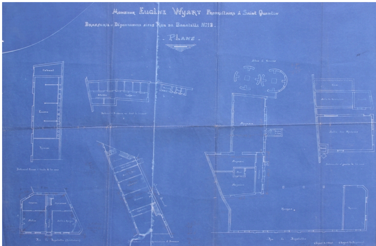
Plans de la brasserie en 1914 (AD Aisne).
