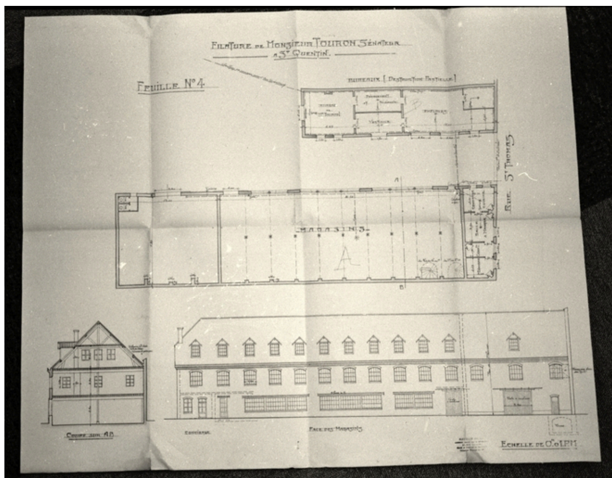
Plan des magasins et bureaux situés à l'entrée du site avant 1914, rue Voltaire, par Nalet : état en 1914 (AD Aisne).
