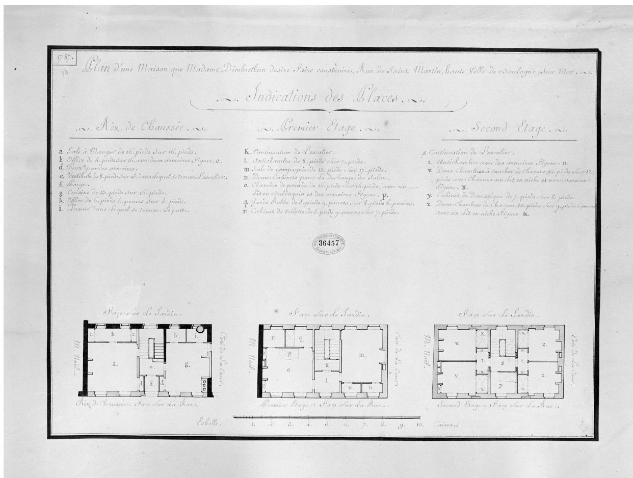
Maison, rue St Martin, 1787 : plans. B.M. Boulogne-sur-Mer, 13e portefeuille, fol. 7.
