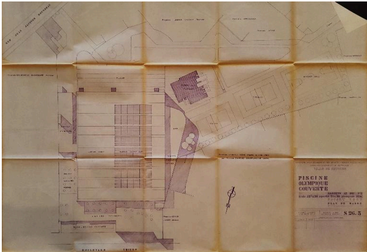
Avant-projet de piscine olympique couverte : plan de masse, André Evard architecte, 1967-1968 (AN ; 19800382/234).
