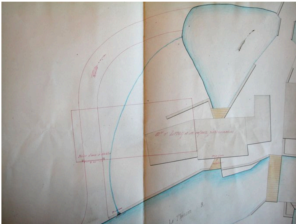
Plan du moulin à foulon Léger-Leroy, annexé à la demande de reconstruction, par Crouzet (garde-rivière), 1855.
