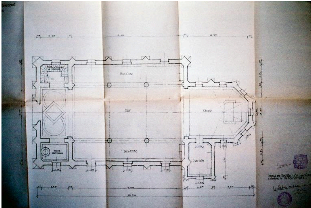
Projet de reconstruction de l'église : plan, Jacques Debat-Ponant (architecte), 16 février 1924 (AD Somme ; 99 O 1468).
