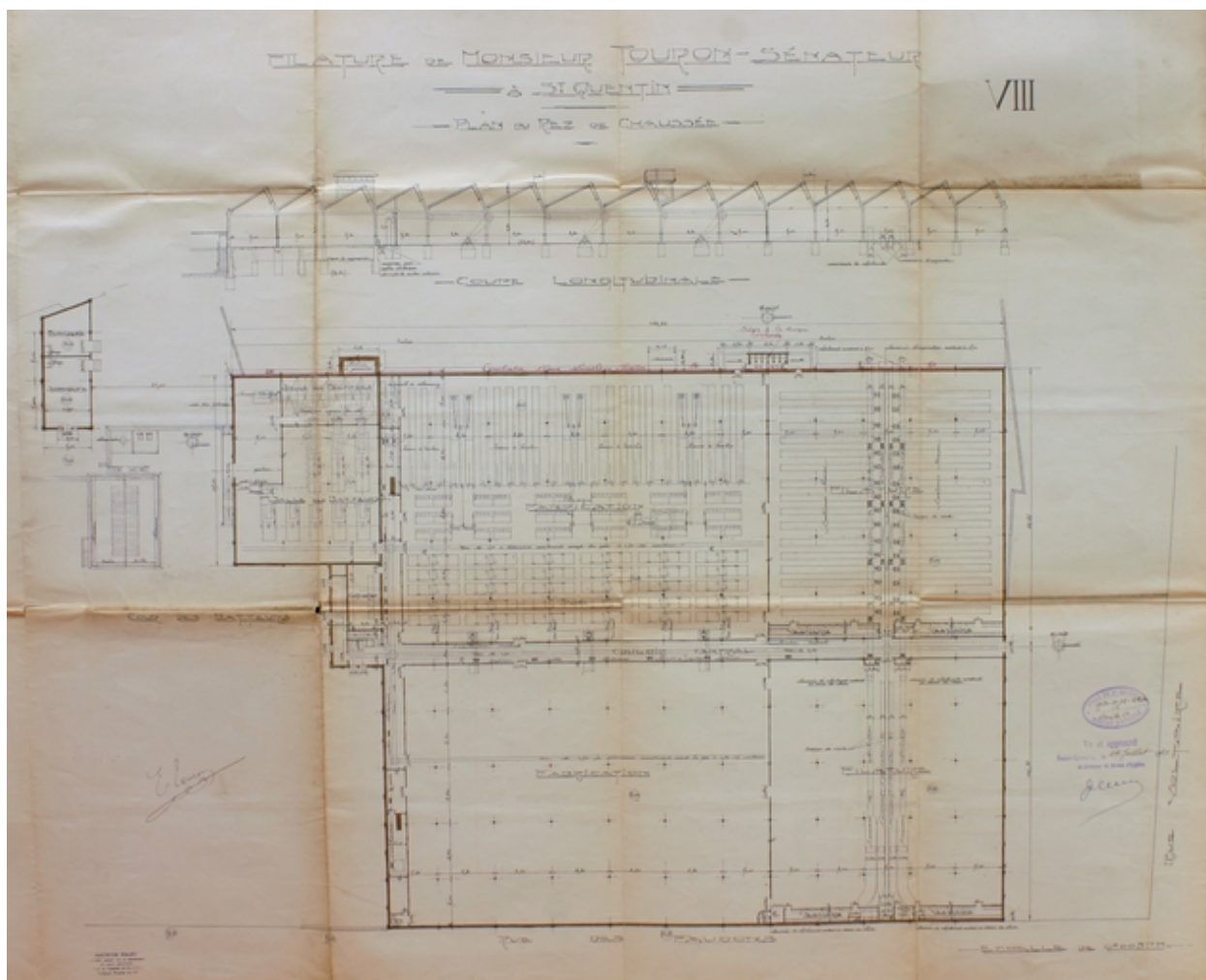
Plan du rez-de-chaussée des ateliers, par Narlet (arch.), 1921 (AC Saint-Quentin).
