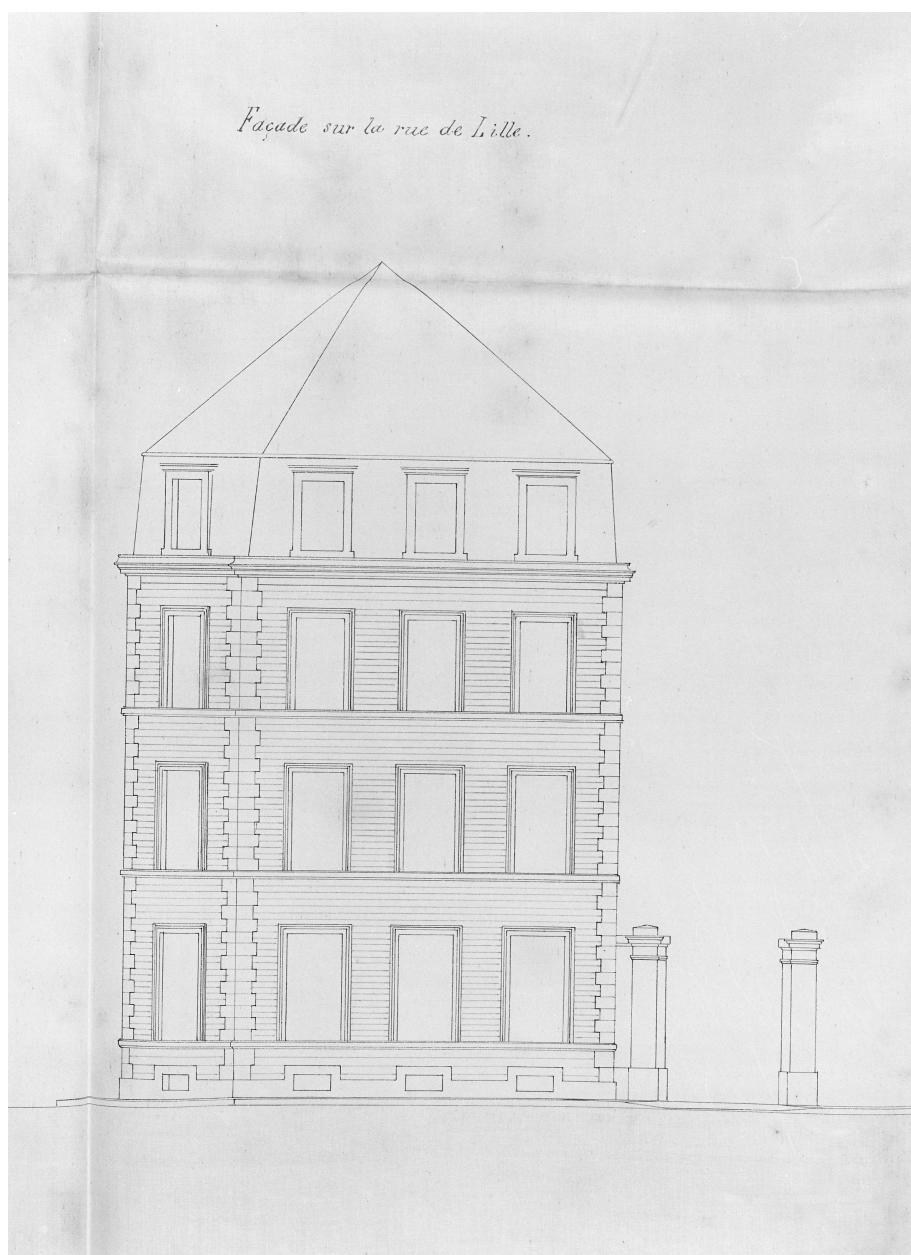
Presbytère, façade rue de Lille, plan (1881). A.D. Pas-de-Calais (2 0 - 1120).
