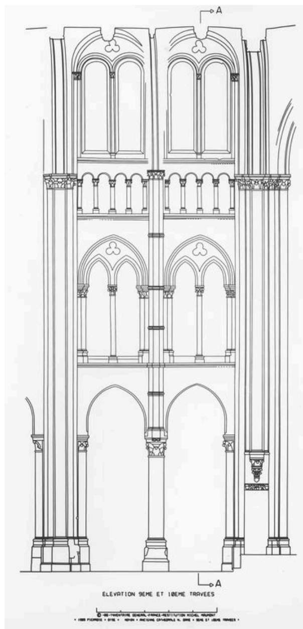
Élévation nord (9e et 10e travées de la nef).
