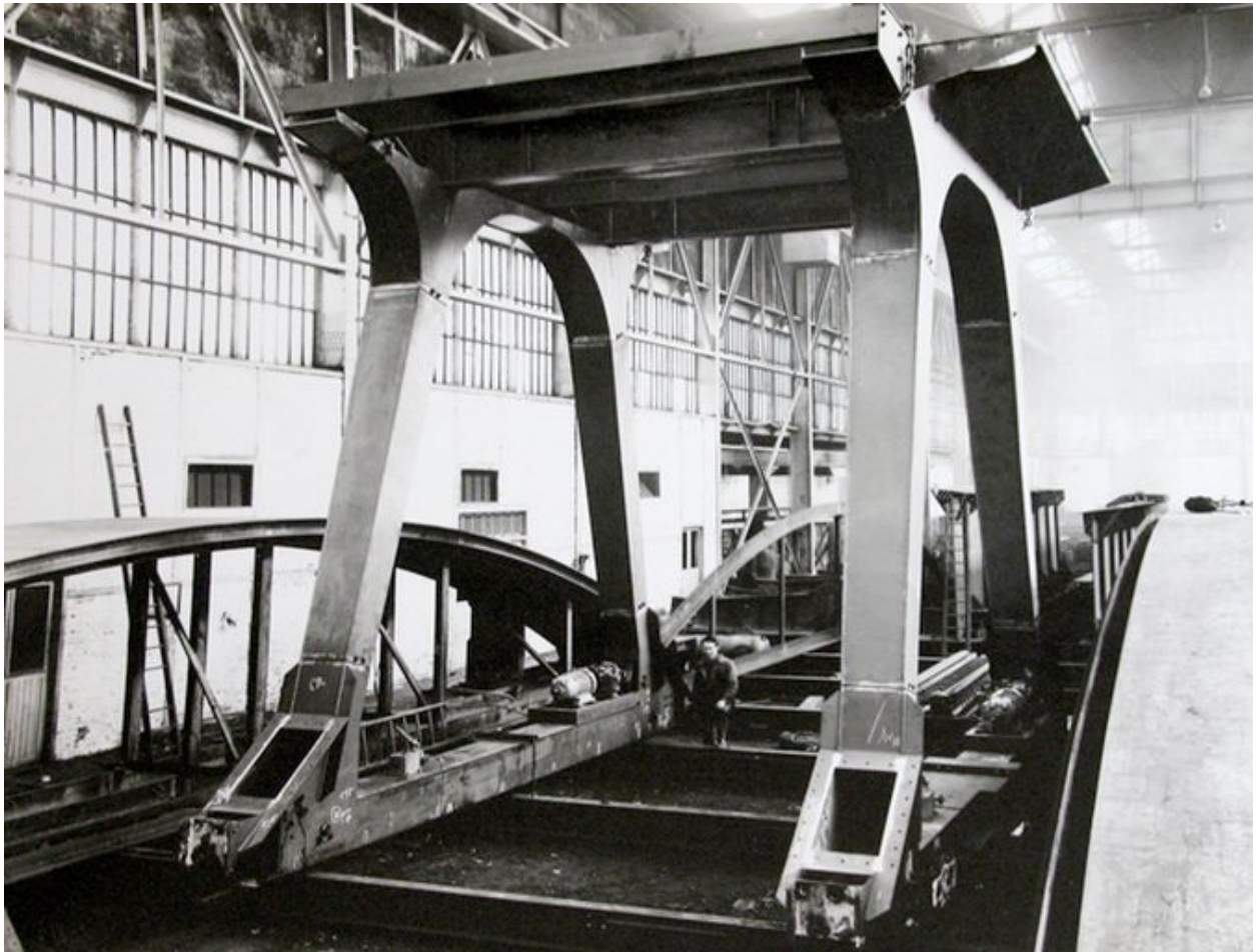
Appareil de manutention construit pour la centrale EDF de Marckolsheim, 1960 (AP).
