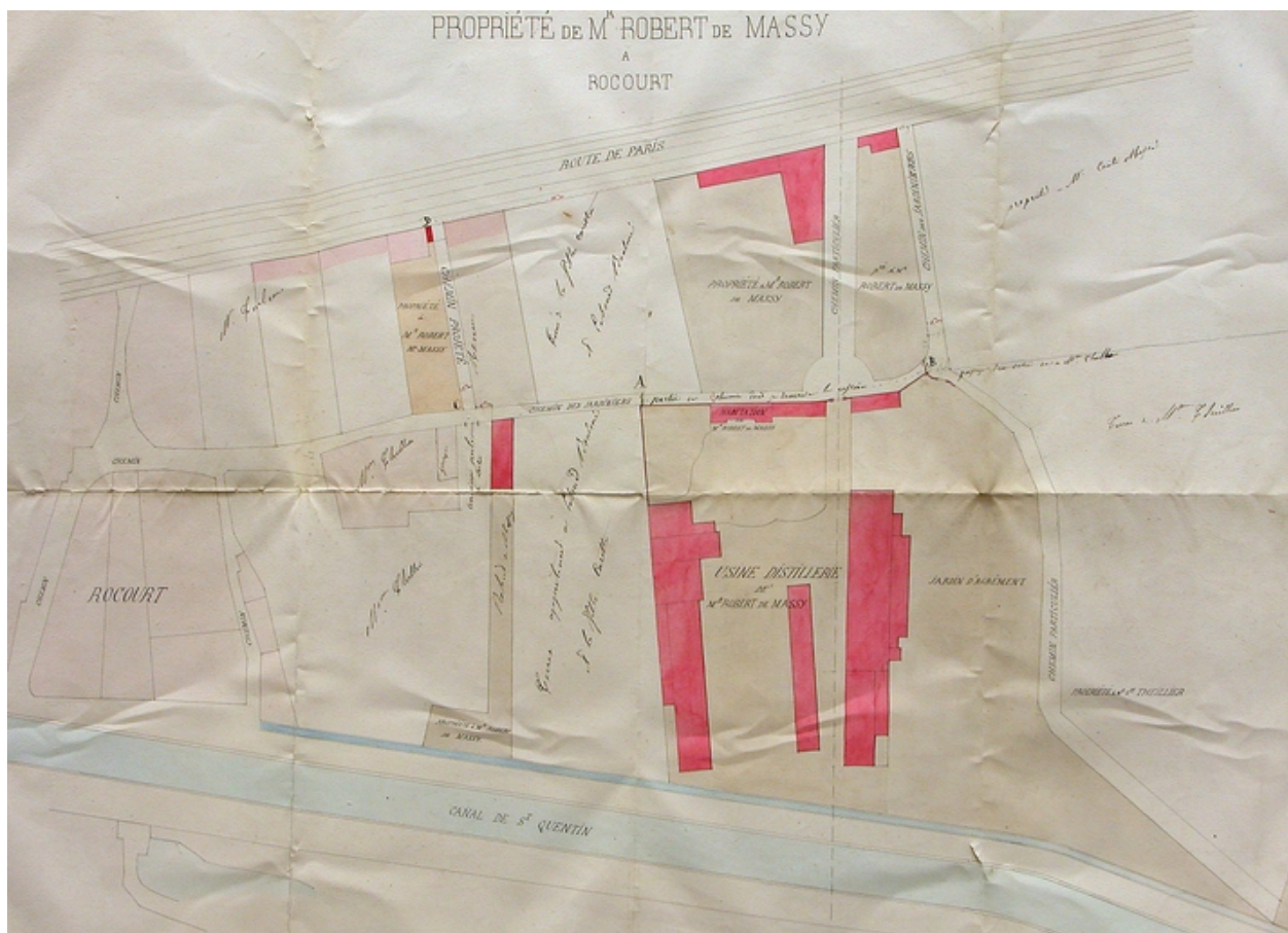
Plan masse de l'Usine de Rocourt, par Schneider, 1857 (AC Saint-Quentin).
