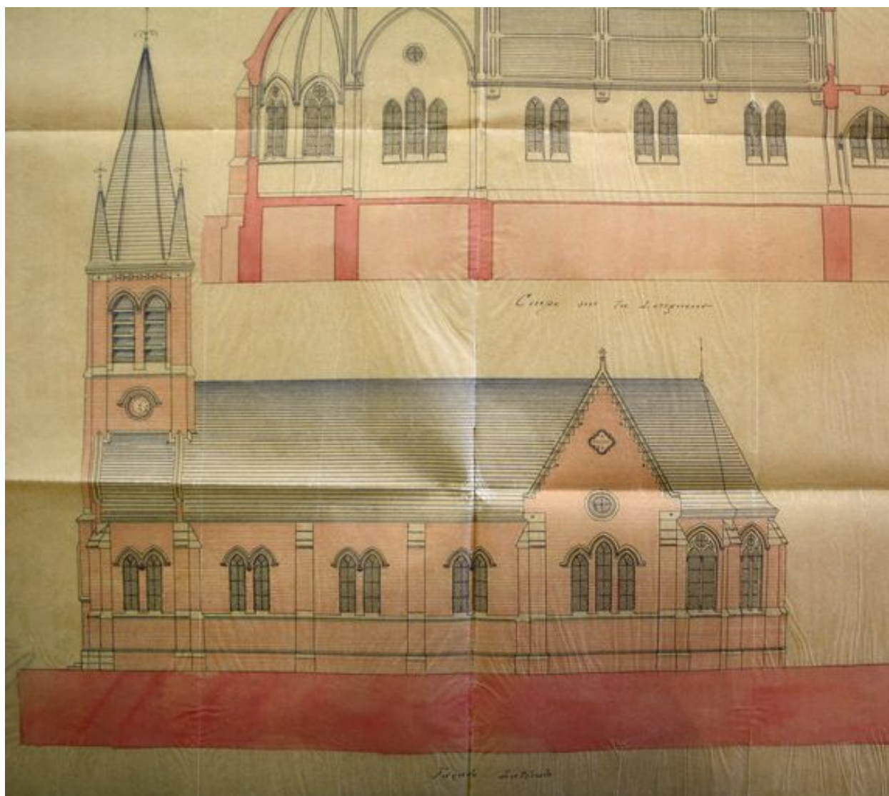
Elévation longitudinale de la nouvelle église, par Herbault (architecte), 1866 (AD Somme ; 99 O 3775).
