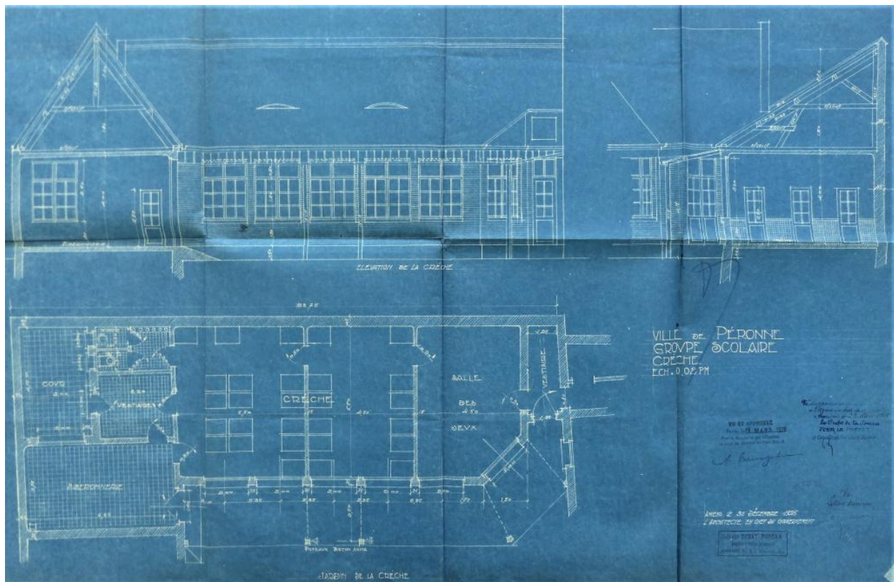
Ville de Péronne. Groupe scolaire. Crèche. Plan au sol, élévation et coupe, Jacques Debat-Ponsan architecte, 1925 (AD Somme ; 99O 3002).
