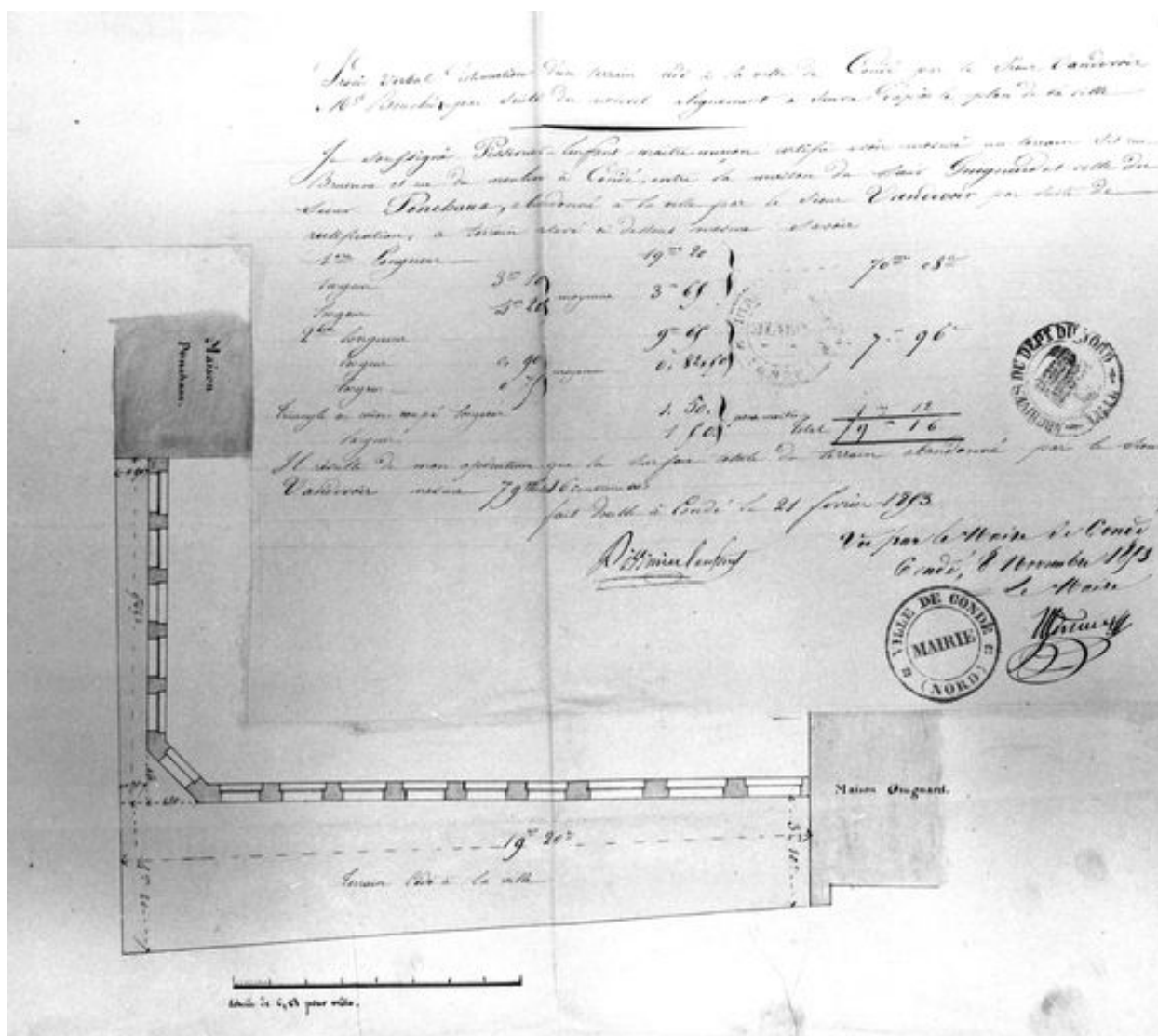
Proçès-verbal de mesure du terrain cédé à la ville par le sieur Vandevor lors de la reconstruction de son immeuble : plan au sol, 1853 (AD Nord).
