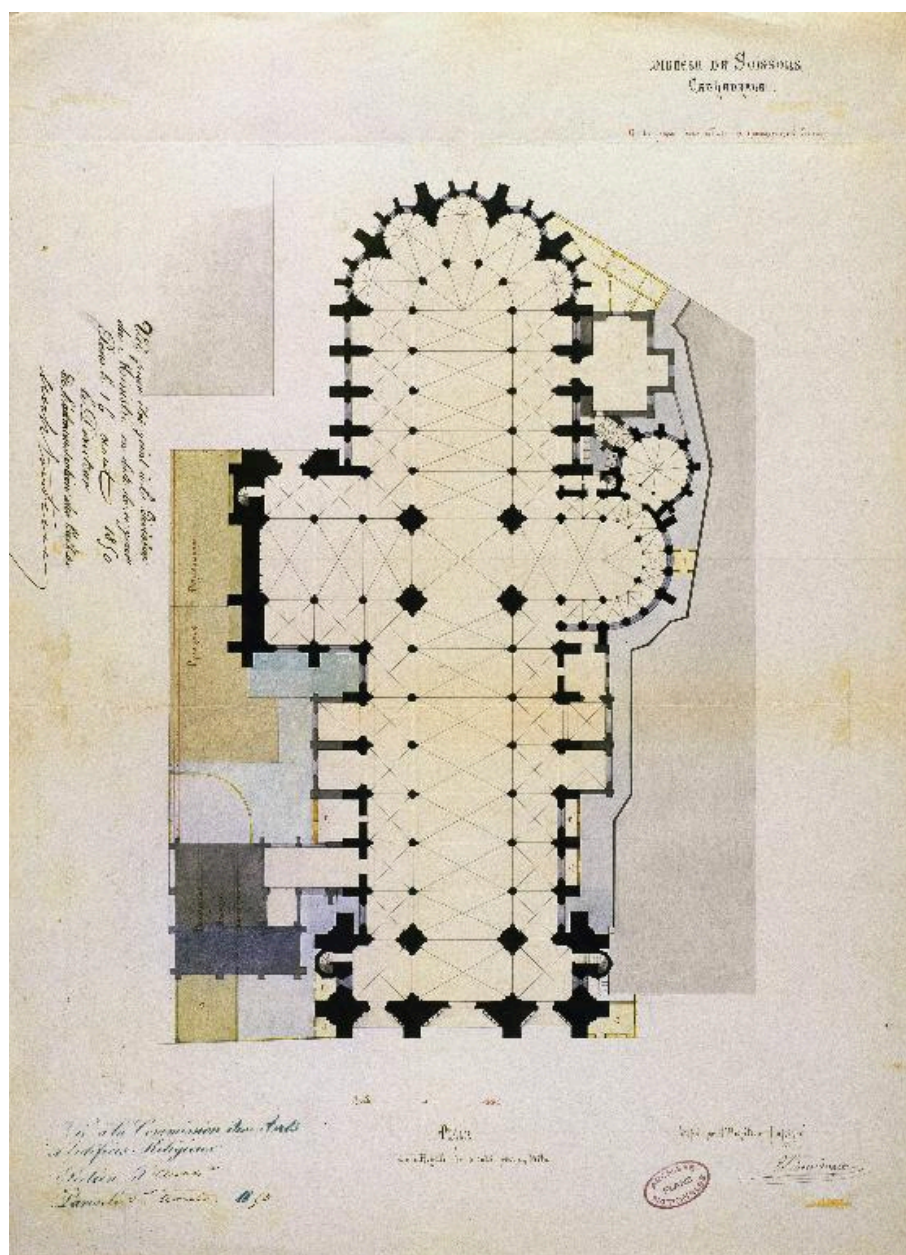
Plan de la cathédrale, dressé en 1850 par l'architecte Émile Boeswillwald, portant l'indication de constructions adjacentes à démolir (AN : F 19 7887).
