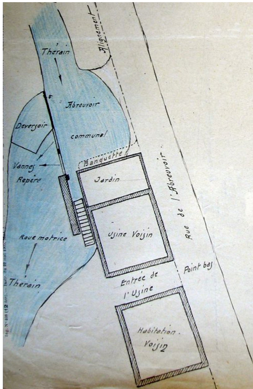
Plan détaillé de l'usine Voisin, Bouloche (ingénieur des Ponts-et-Chaussées), 8 février 1928.
