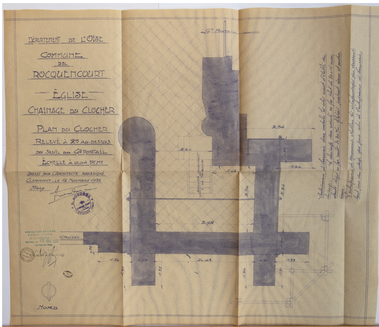
Rocquencourt. Plan du clocher à 2 m au-dessus du seuil du grand portail, architecte Boudoux, 1937 (AD Oise).
