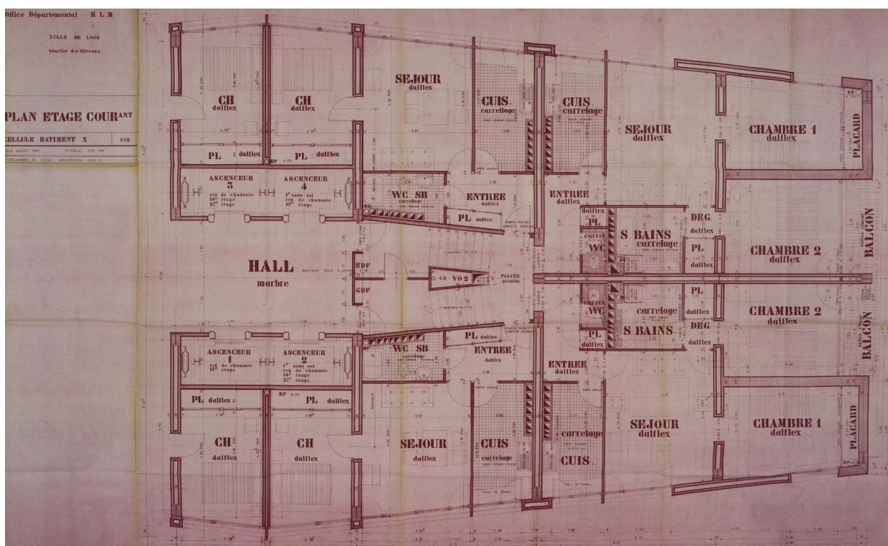
Plan détaillé d'une cellule d'un étage courant de la tour Kennedy, juin 1963, F.-P. Delannoy et J.-P. Secq (arch.) (AD 59 ; 1465 W 66).
