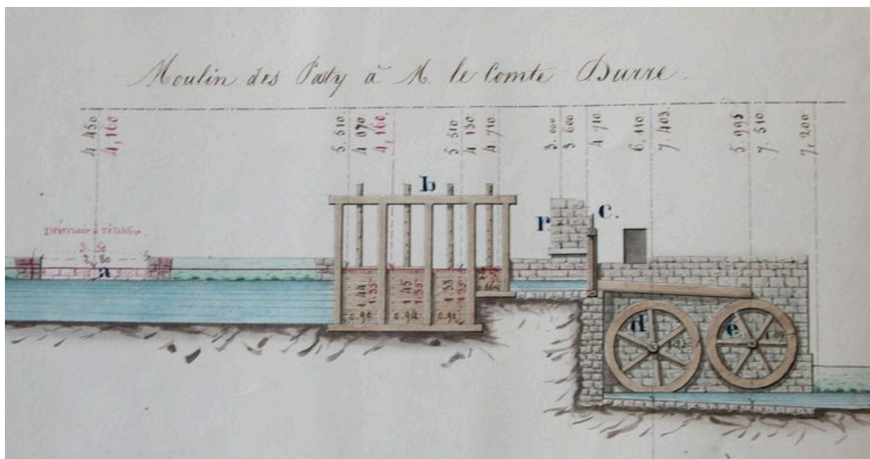
Profil du moulin des Pâtis à Mr le comte Durre, annexé au projet de règlement des moulins de Thérines, détail, 24 novembre 1837.
