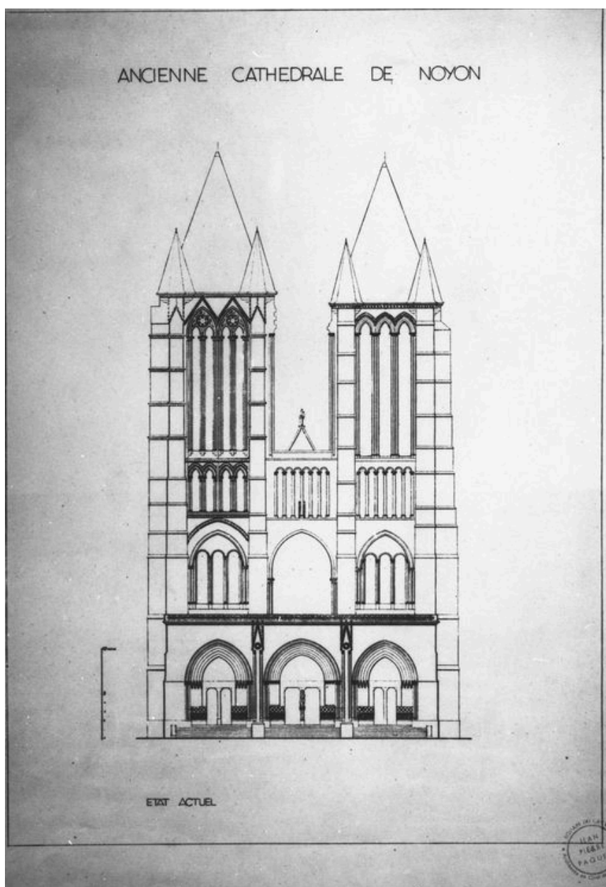
Elévation ouest, état actuel. Relévé par Paquet 1948-1950.
