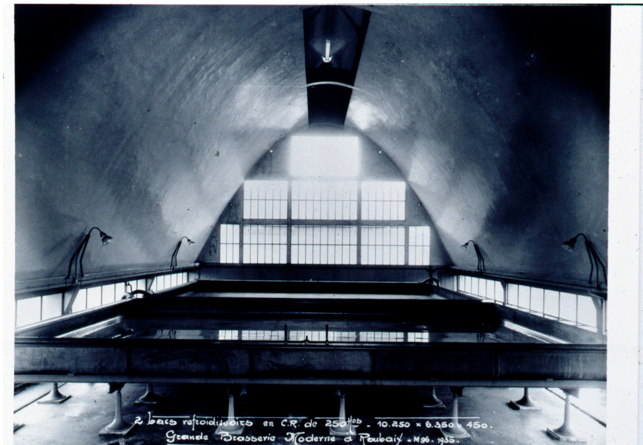
Bacs refroidisseurs (AP Coutances).
