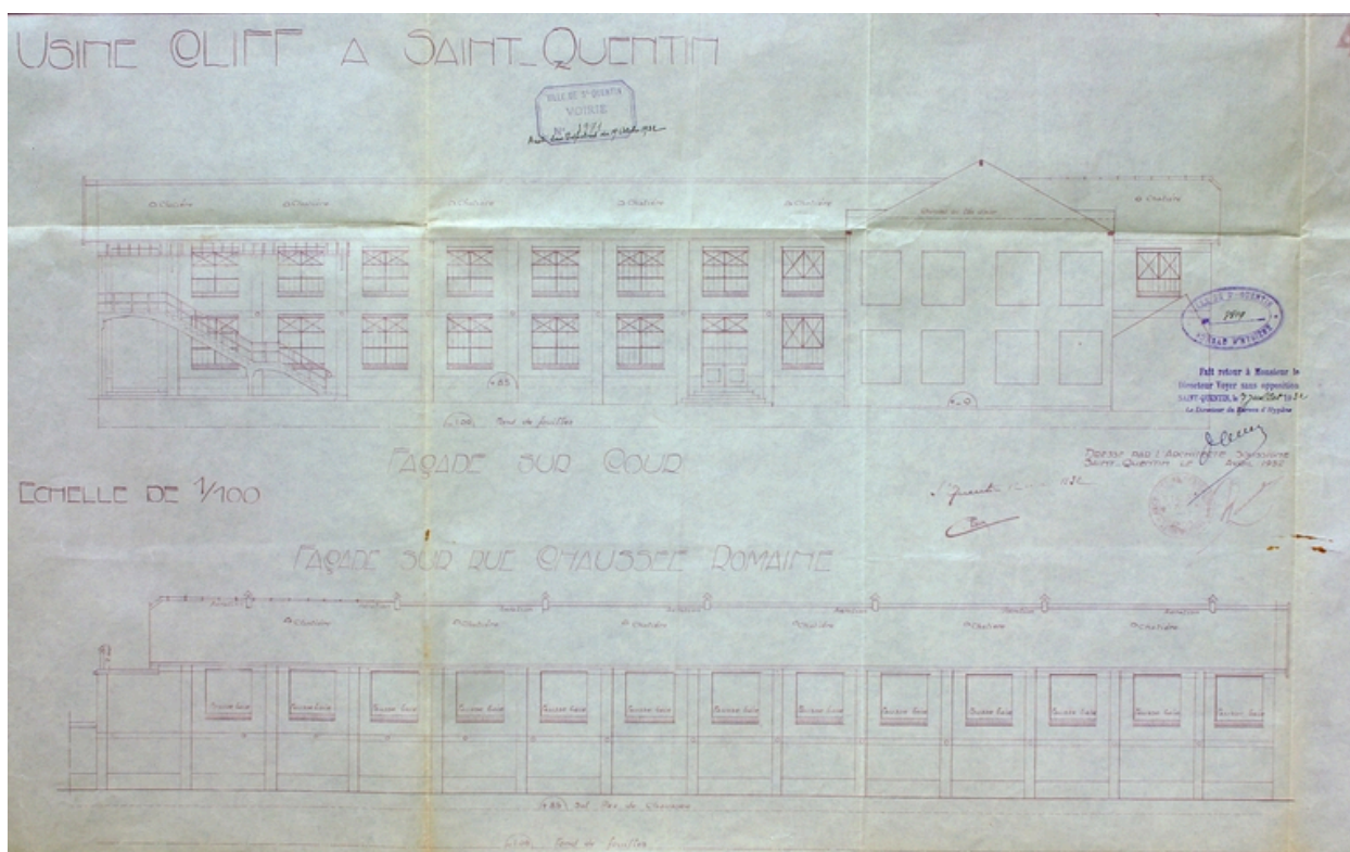
Plan et élévation par Antoine, Boyer et Lacouture : construction d'un atelier en 1932 (AC Saint-Quentin).
