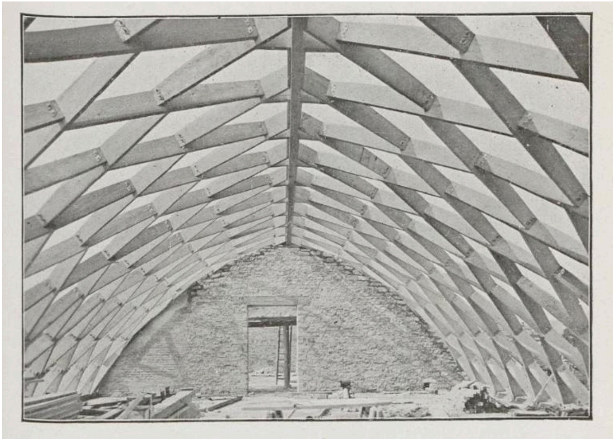
La halle en construction. Extrait de CRESTIN, F. "Les charpentes à lamelles en bois". Revue des eaux et forêts : économie forestière, reboisement, 1941.
