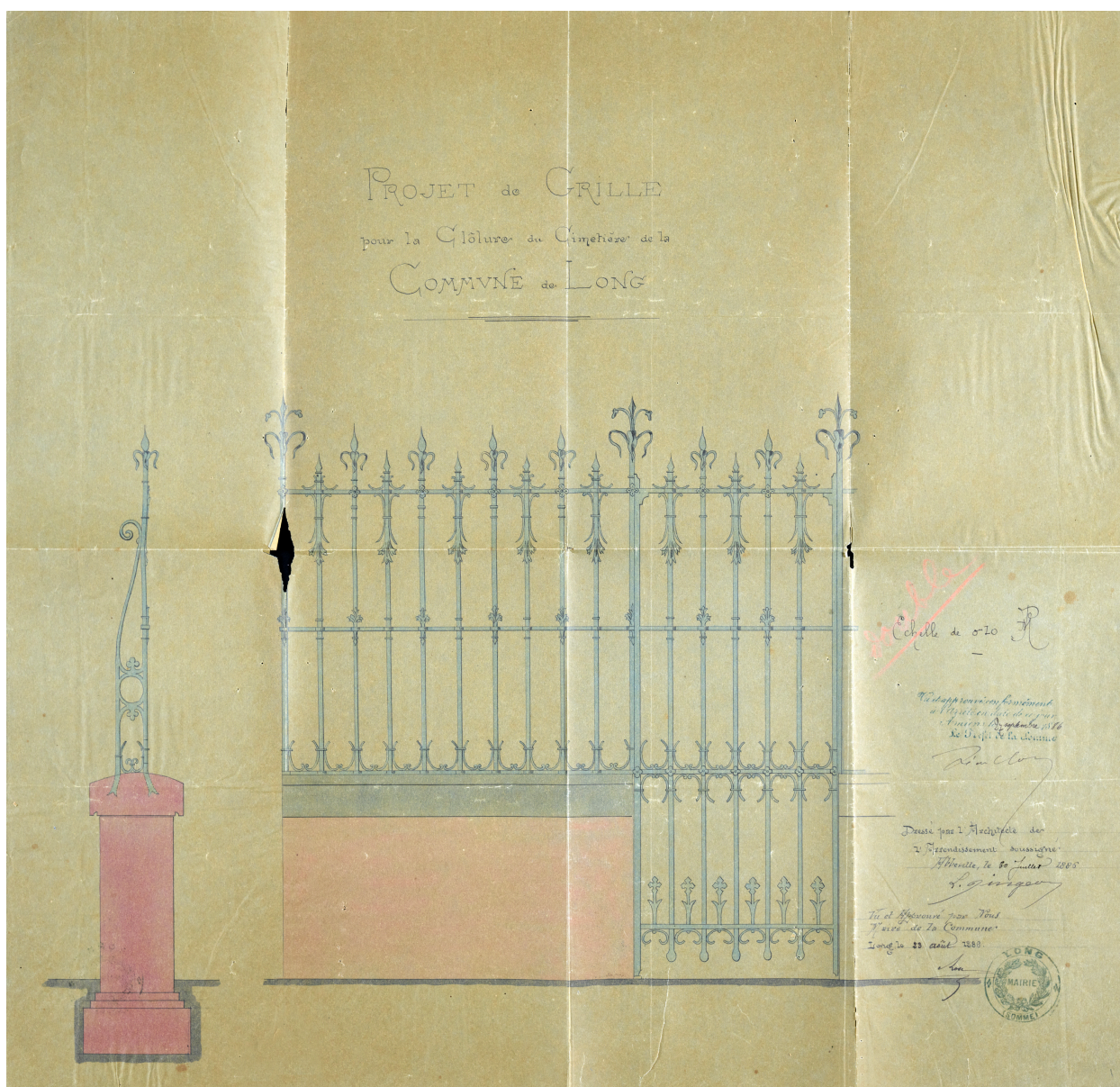
Projet de grille pour la clôture du cimetière, par Léopold Digeon, 30 juillet 1886 (AD Somme ; 99 O 2380).
