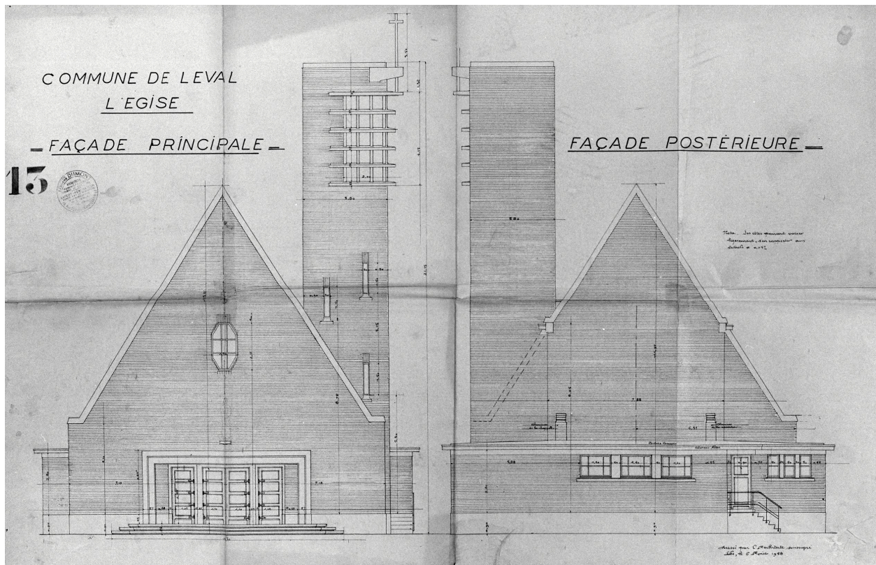
Élévations antérieure et postérieure de la nouvelle église. Plan de Fernand Dumont (architecte communal), 6 août 1958 (AC Leval ; dossier église).
