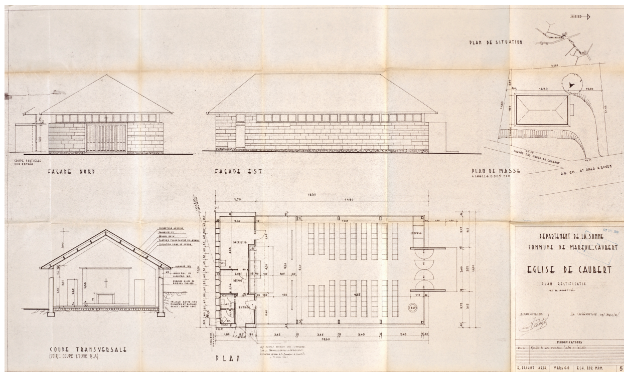
Église de Caubert, plan, élévation et coupe, par Roger Pachot, architecte, mars 1960 (AD Somme ; 1272 W 57).
