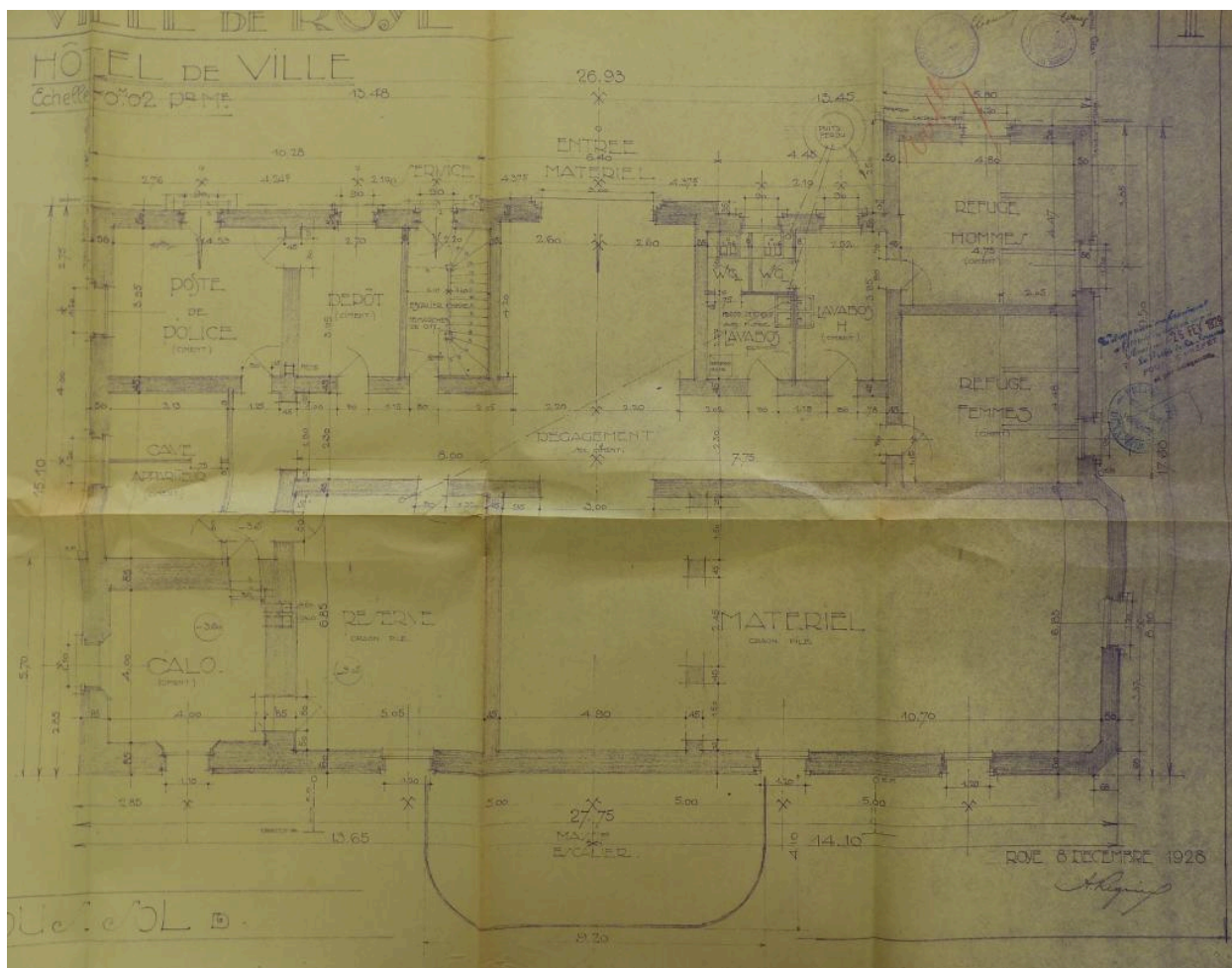
Ville de Roye. Hôtel de ville. Plan du sous-sol. A. Régnier architecte, 1928 (AD Somme ; 990 3296).
