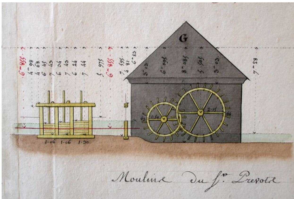
Profil d'élévation du moulin appartenant au sieur Prévost, 1812.
