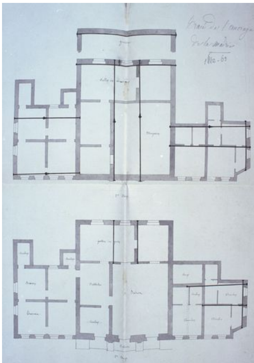
Tracé de l'ancrage de la mairie, plans des premier et deuxième étages, 1862-63 (Archives municipales de Condé-sur-l'Escaut).
