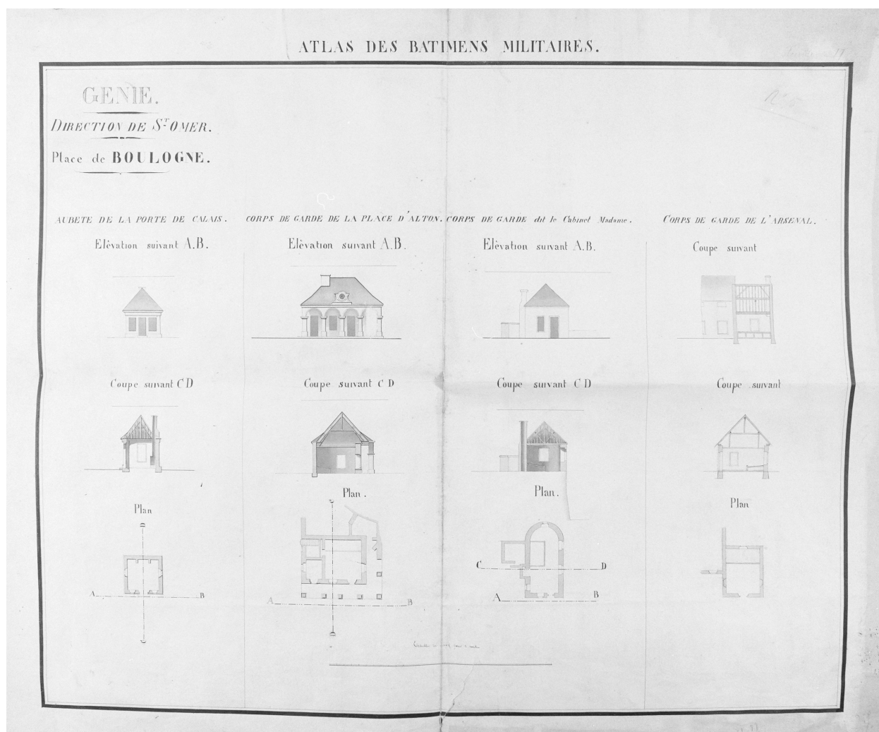
Aubète, plan, coupe, façade. Atlas des bâtimens militaires, Génie, direction St Omer, place de Boulogne (collection privée).
