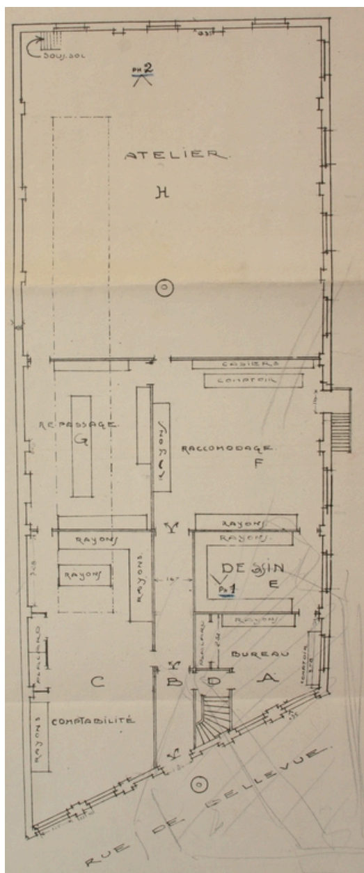
Plan d'ensemble des ateliers avant les destructions de la Première Guerre mondiale, dressé, par Briault, 1919. Détail. (AD Aisne).
