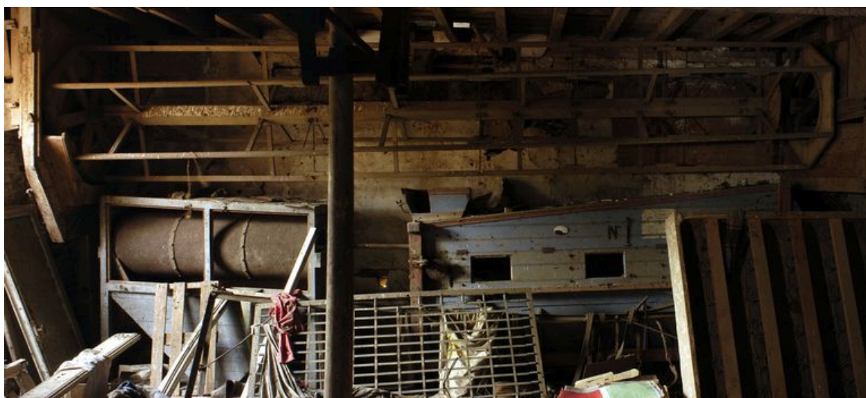
Vue d'ensemble du bluttoir et du sasseur.
