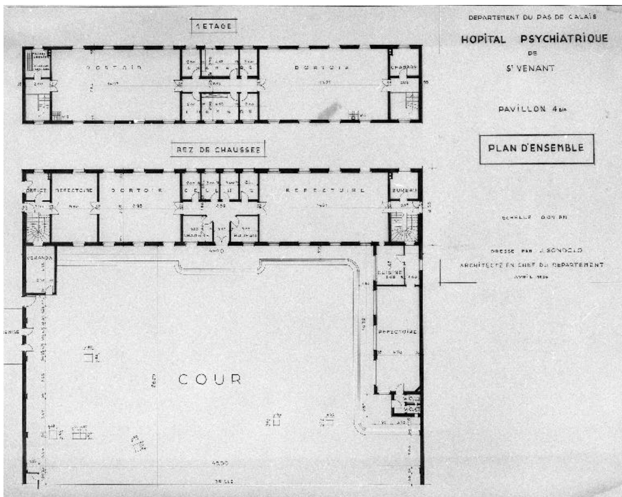
Bâtiment d'hospitalisation dit pavillon 4 bis, plan de distribution du rez-de-chaussée et du 1er étage par l'architecte Gondolo, avril 1956, vue d'ensemble (AD Pas-de-Calais).
