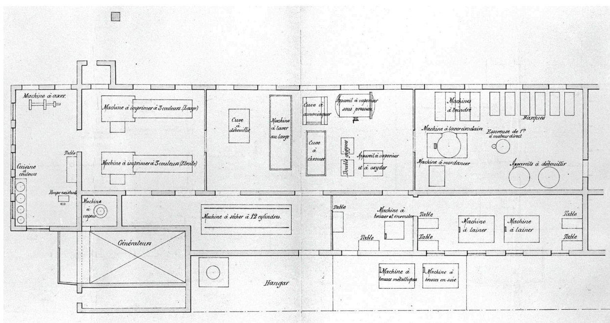
Piequet. Installation d'une teinturerie. Plan masse, 1891 (AD Nord ; M4172930).
