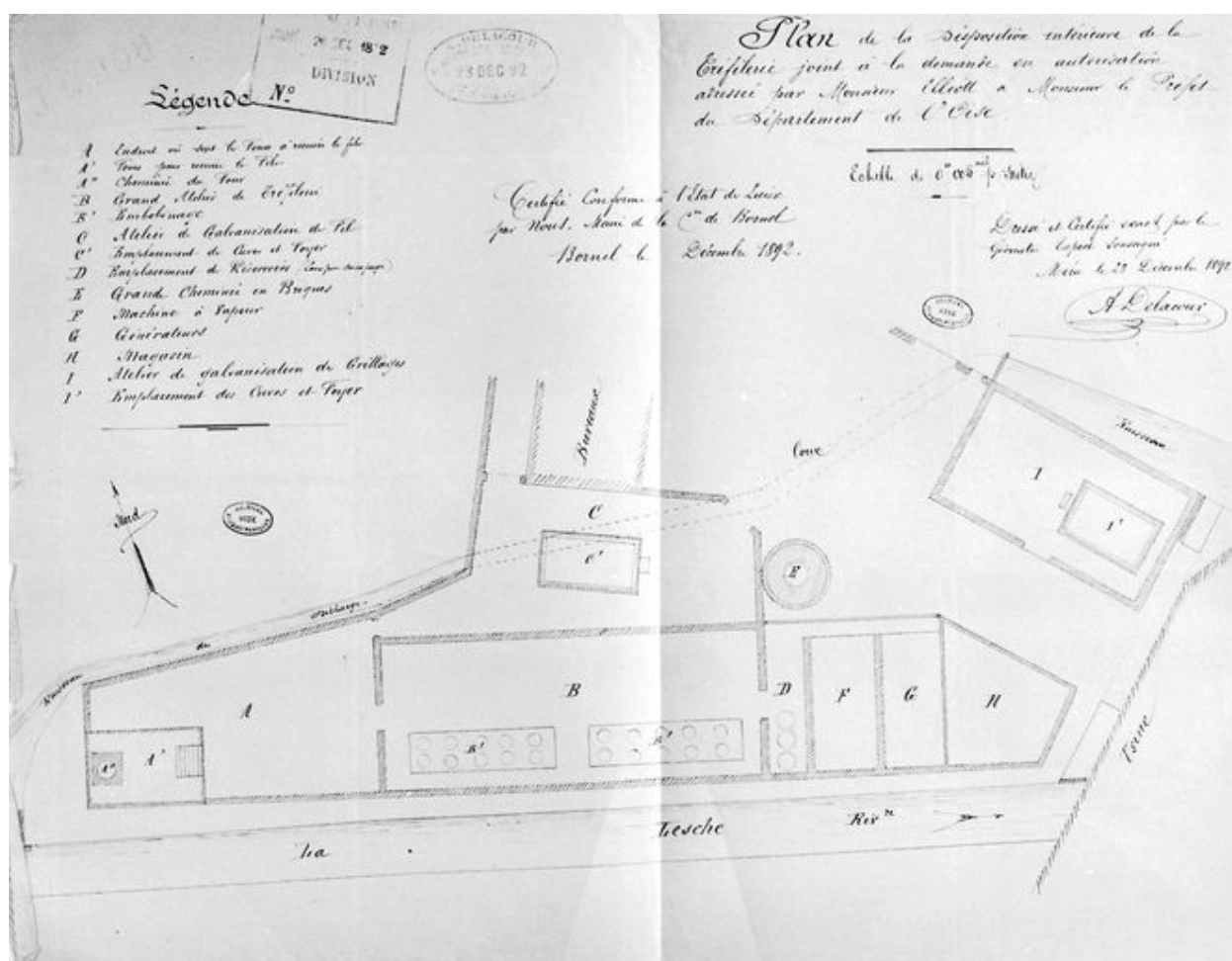
Plan de détail de la tréfilerie Elliot, 1892 (AD Oise ; Mp 2426).
