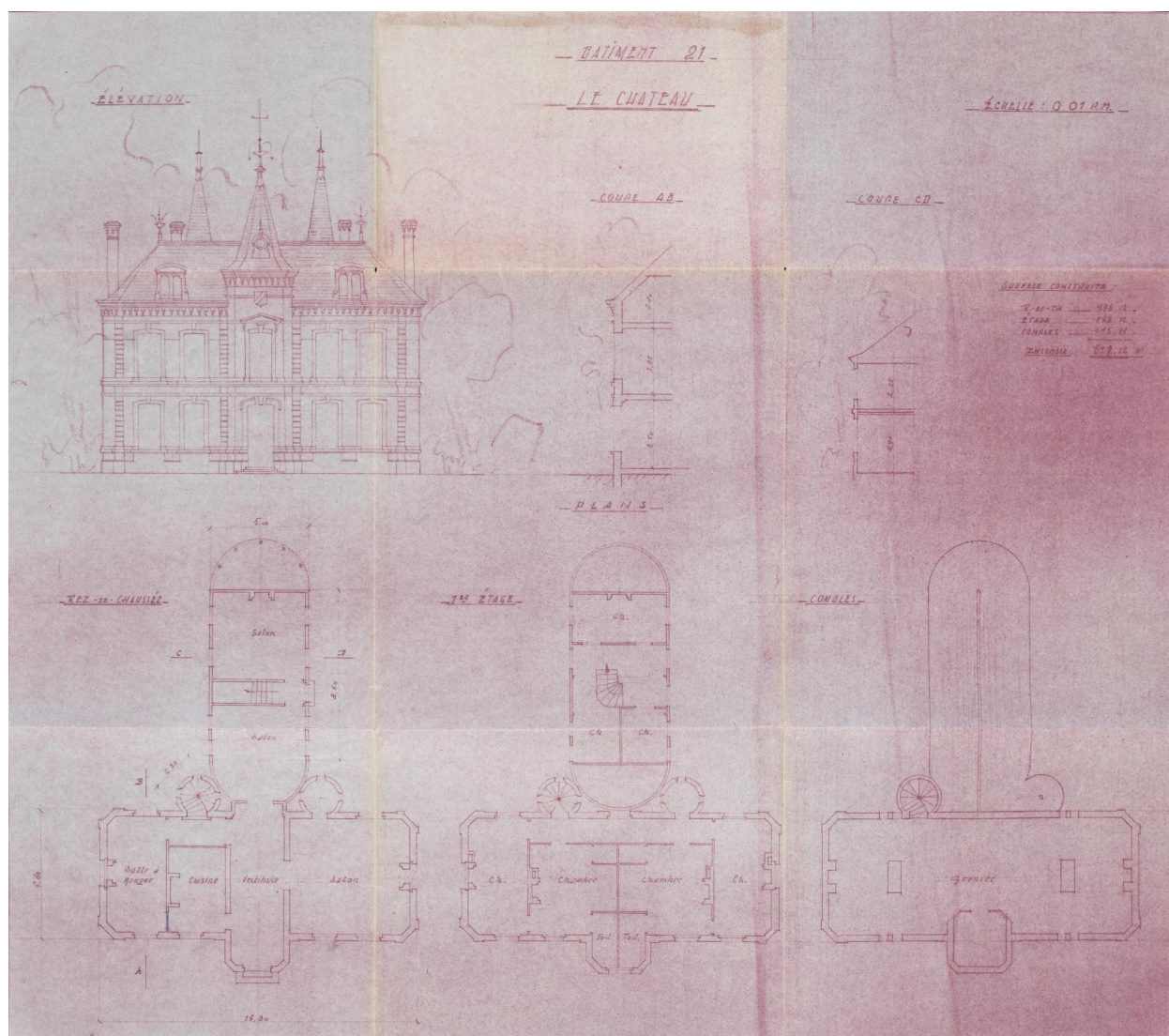
Plan et élévation de la demeure, dressé par l'architecte Roger Pachot, [s.d.] (AD Somme, 1275 W 103).
