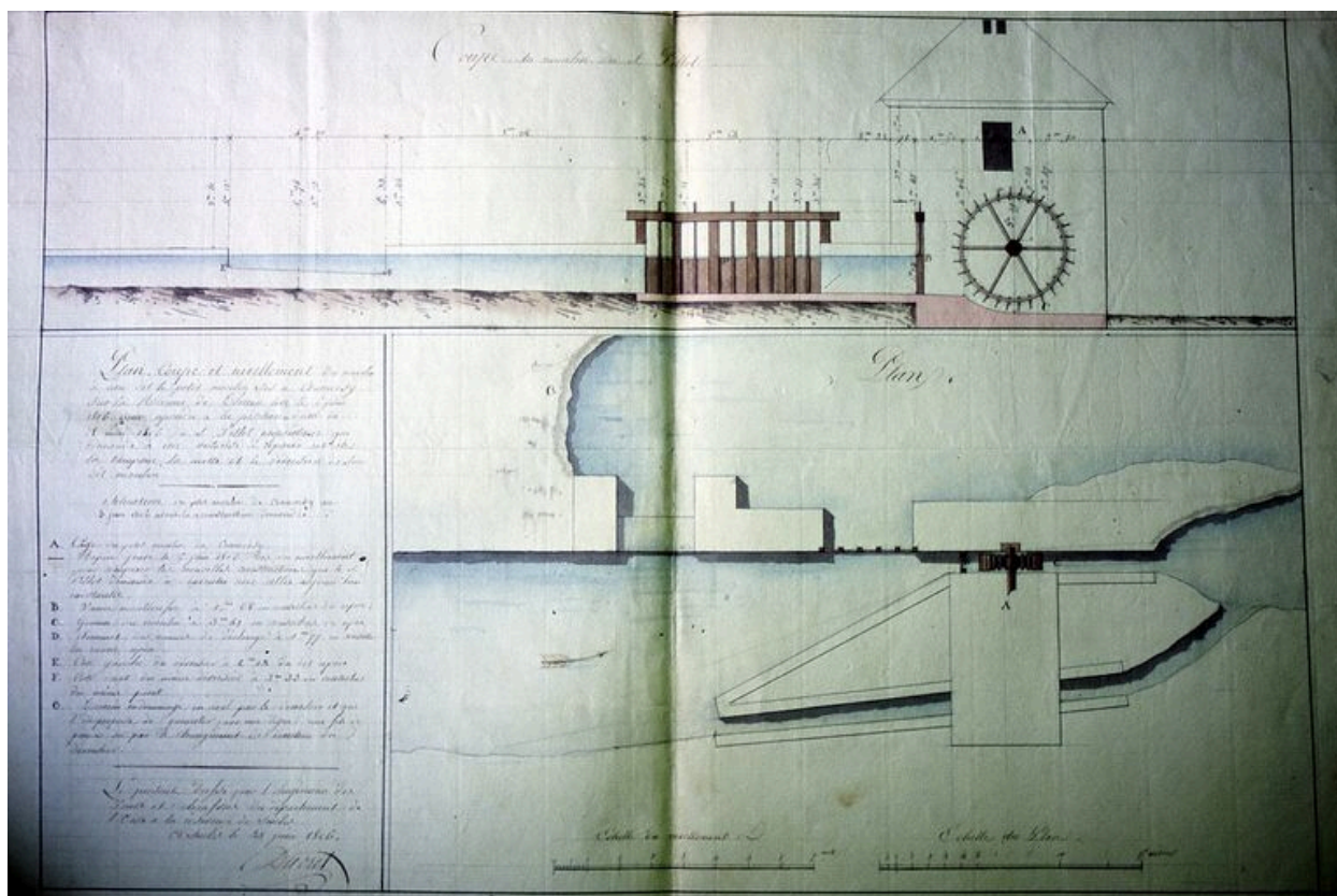
Plan et coupe du Petit Moulin de Cramoisy, 1806.
