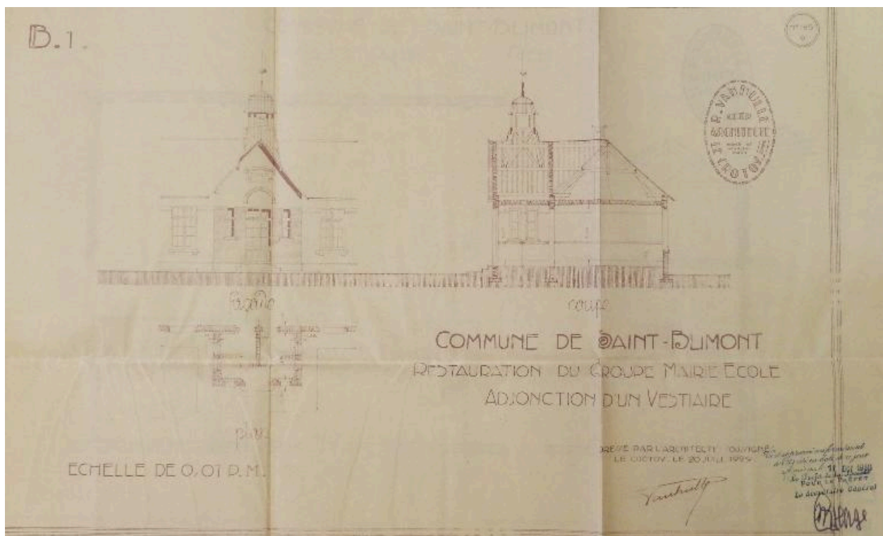
Coupe et élévation du vestiaire, 1930 (AD Somme ; 99 O 3366).
