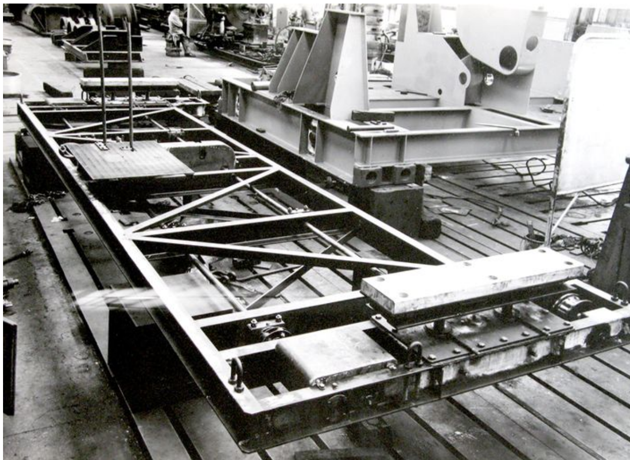
Lorry de stockage des batardeaux. Centrale EDF de Marckolsheim dans le Bas-Rhin (AP).
