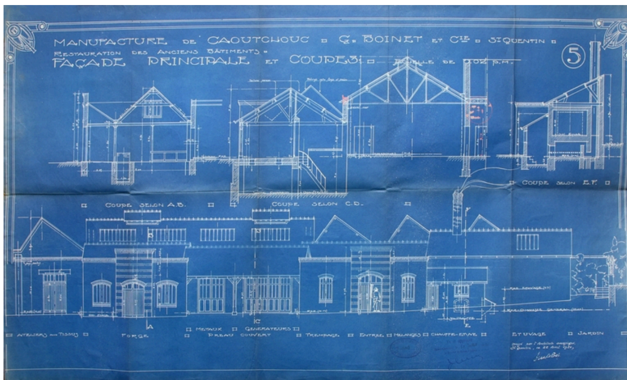
Façade antérieure des ateliers et coupes, par Le Bot, 1920 (AC Saint-Quentin).
