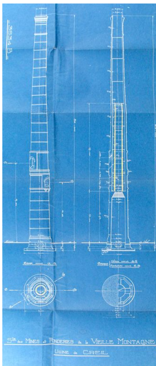
Plan des cheminées construites en 1923 (AD Oise ; 5Mp2457).
