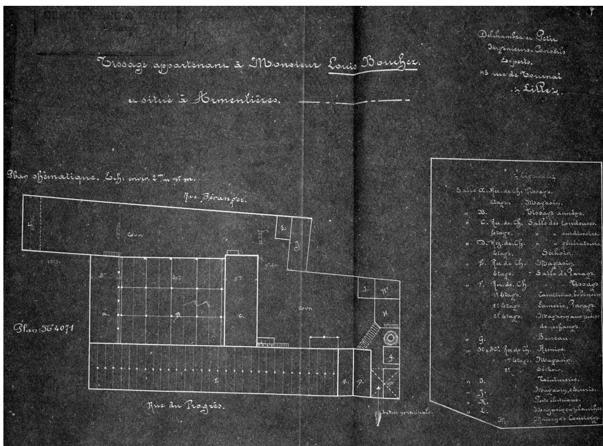
Tissage Louis Bouchez. Office de Reconstitution Industrielle (ORI). Plan masse, avant 1914 (AD Nord ; 10 R 4354).
