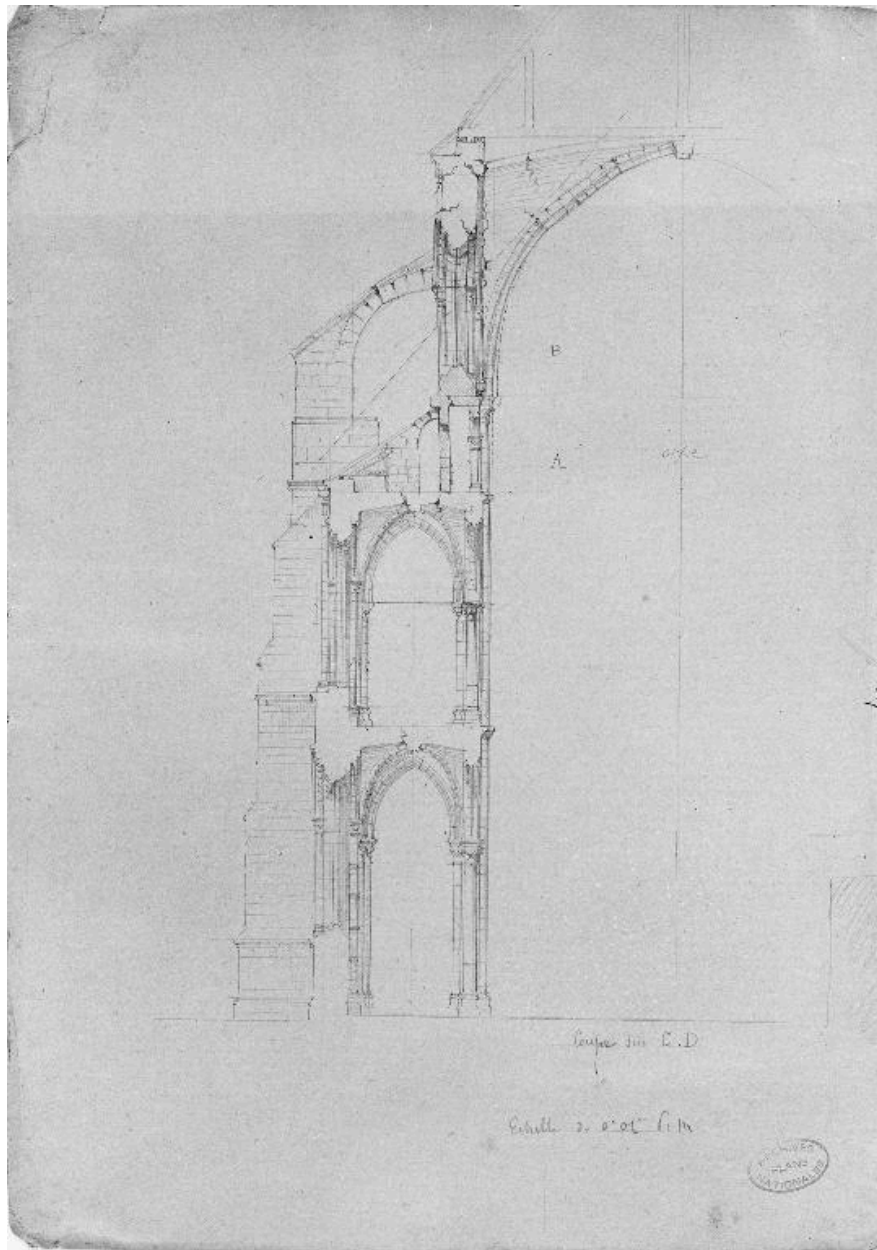
Coupe du bras sud du transept, dessinée vers 1875 par un architecte diocésain dans le cadre de sa restauration (AN : F 19 7888).
