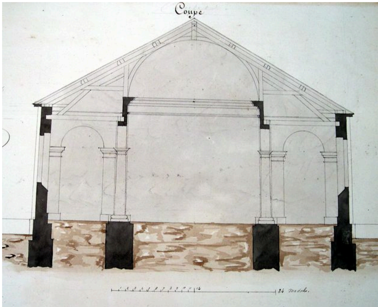
Coupe, par Cheussey, 1846 (AD Somme ; 2 V 18).
