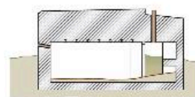
COUPE LONGITUDINALE A-A
