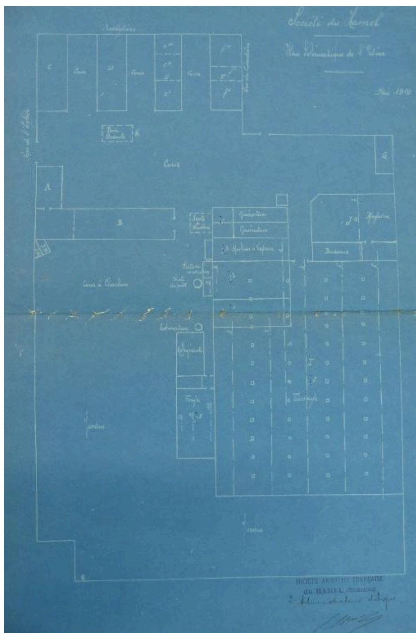
Société du Hamel. Plan schématique de l'usine,1919 (AD Somme ; 10R 633).
